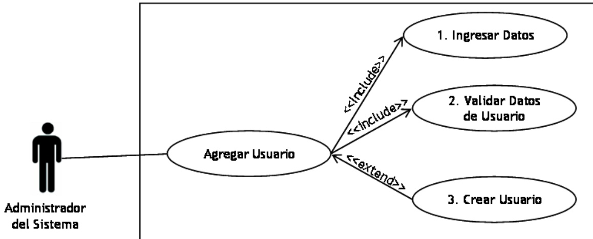
Figura 10. Caso de Uso Agregar Usuario
