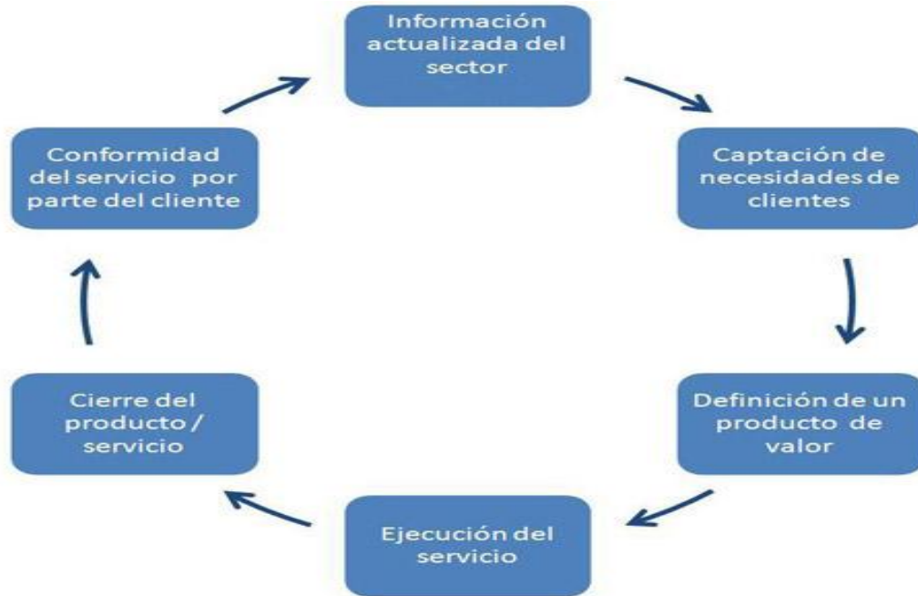
Figura 4. Metodología ADHOC
