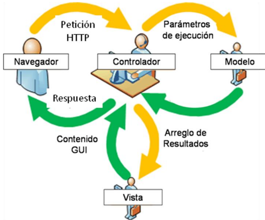
Figura 2. Arquitectura MVC.
