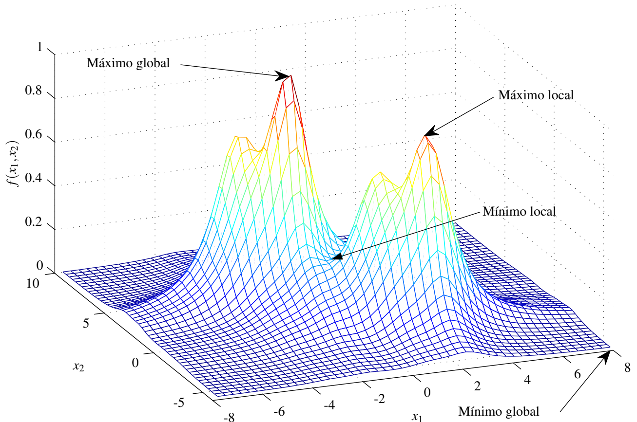
Figura 7.1: Exemplo de função f(x_1, x_2) com ótimo global e local
