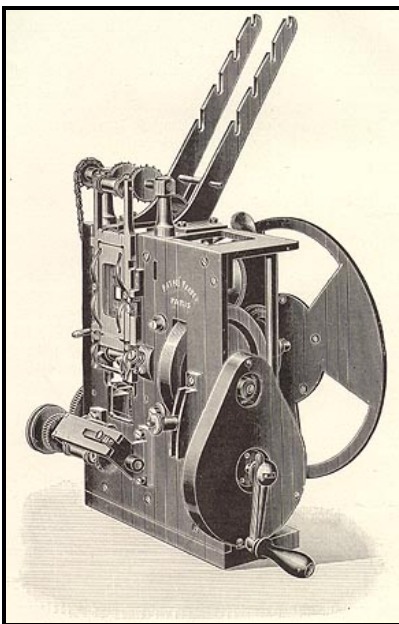
Proyector Pathé modelo 1907
