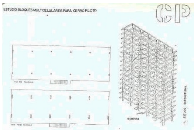
Figura 8. Bermúdez, G. (1954). Plantas elementos standard e isometría estructural Bloque Multicelular CP. Estudio Multicelulares Cerro Piloto CP . Caracas
