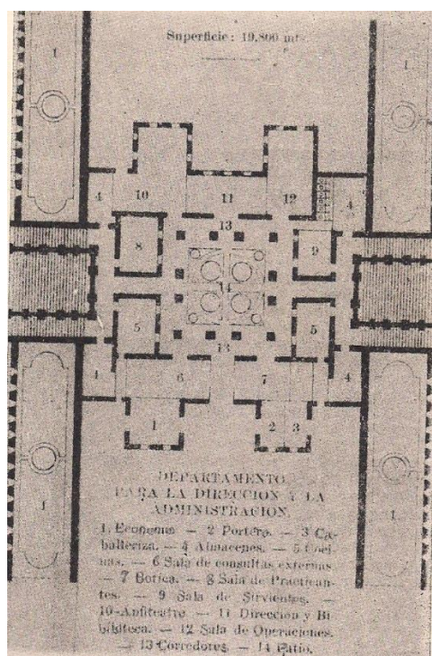
GRAFICO 3.13. EDIFICO CENTRAL DEL HOSPITAL VARGAS. PLANO. 1891
