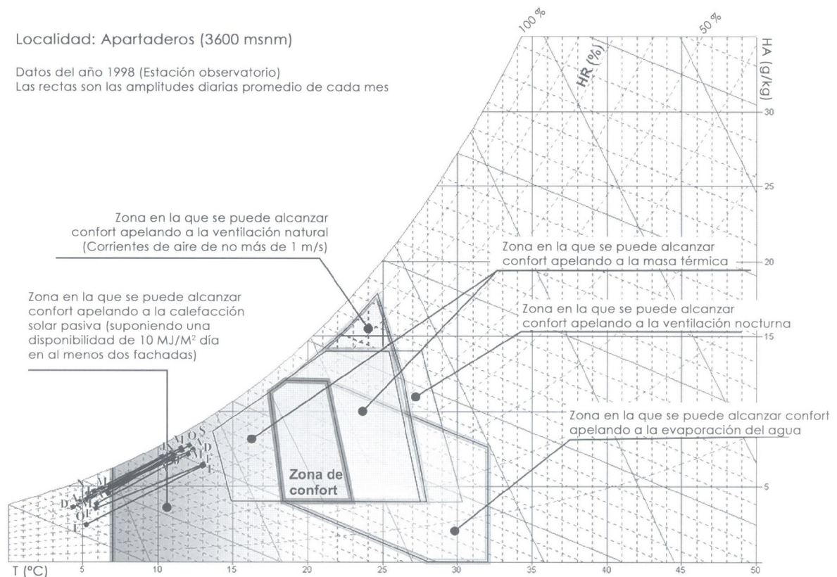
Diagrama 8 Diagrama bioclimático de Apartaderos (zona climática 6)
